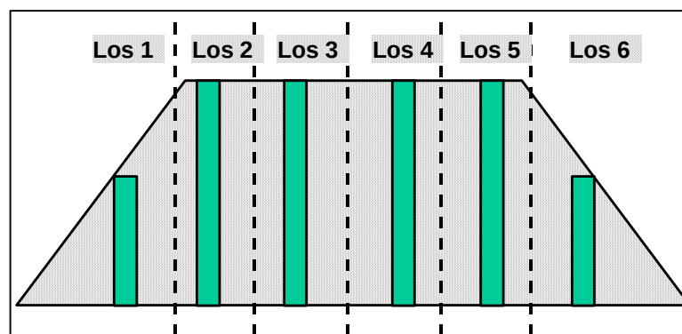
Abb. 4: Schürfschlitten bei trapezförmigen Haufwerken
